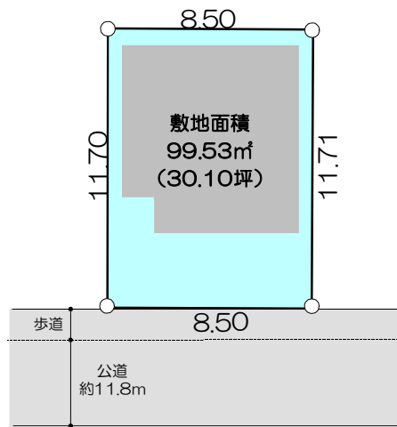
PLAN/区画図
